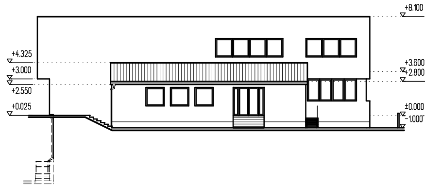
POHLED SEVEROZÁPADNÝ
