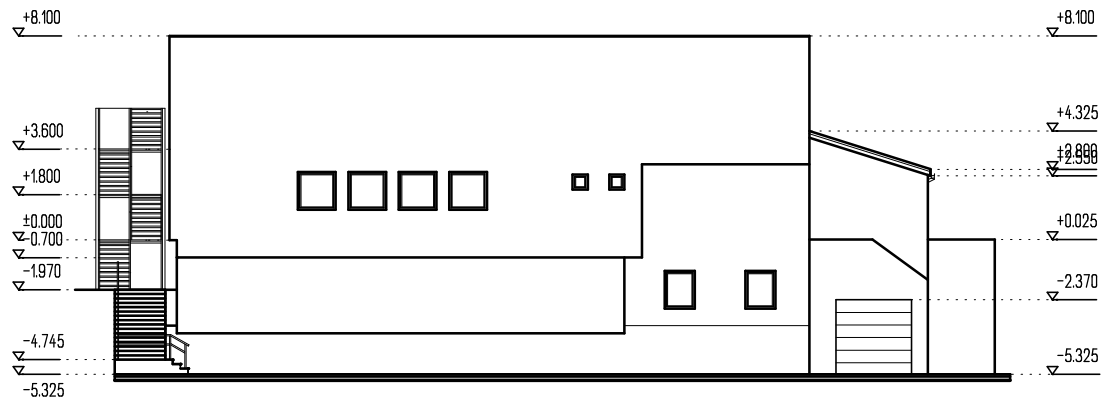
POHLED SEVEROVÝCHODNÝ
