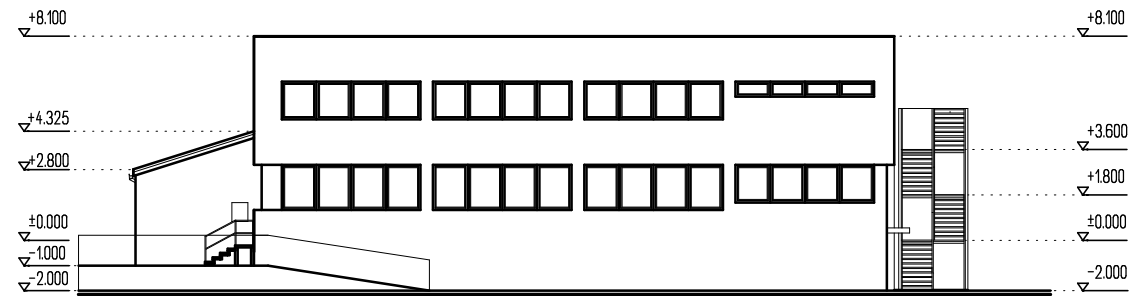
POHLED JUHOZÁPADNÝ
