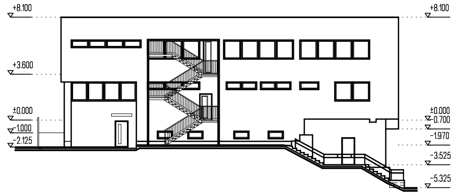
POHLED JUHOVÝCHODNÝ
